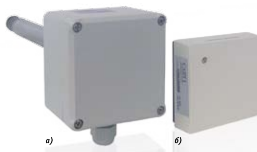
Рис. 4. Датчики качества воздуха Carel: а) ASDQ, б) ASWQ
